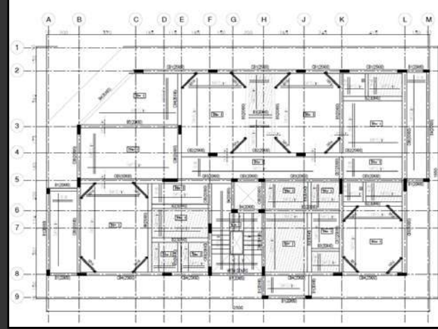
التصميم الإنشائي
